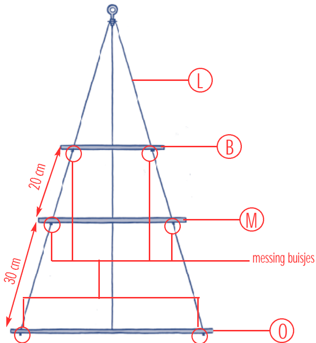
3. plaatsing ringen
