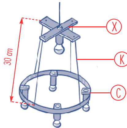
8. ophangen van de lampen
