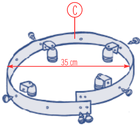
6. ring en fittingen met haakse beugel
