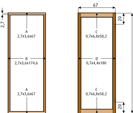
Tekening 2 Binnenframe
