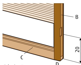
Tekening 4 Detail Frame
