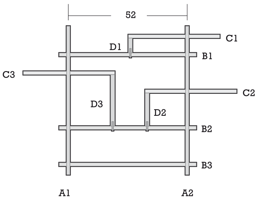
Tekening 2 (maten in cm)
